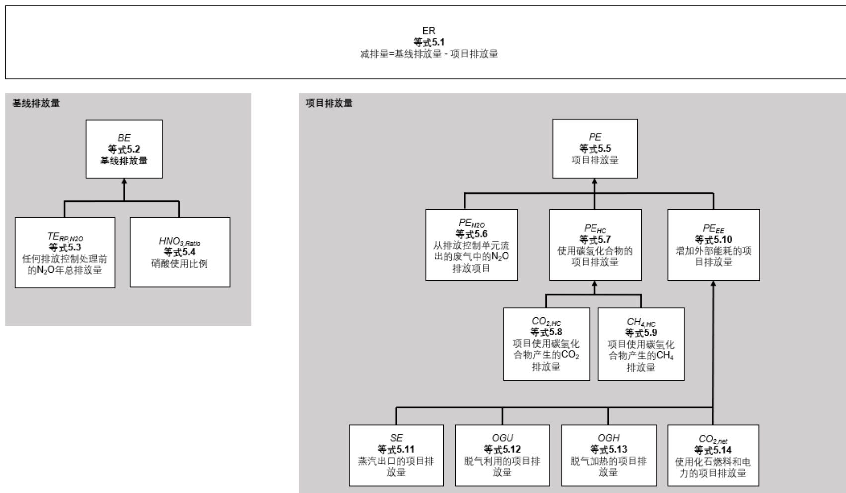
图5.1. 己二酸项目等式组织结构图
